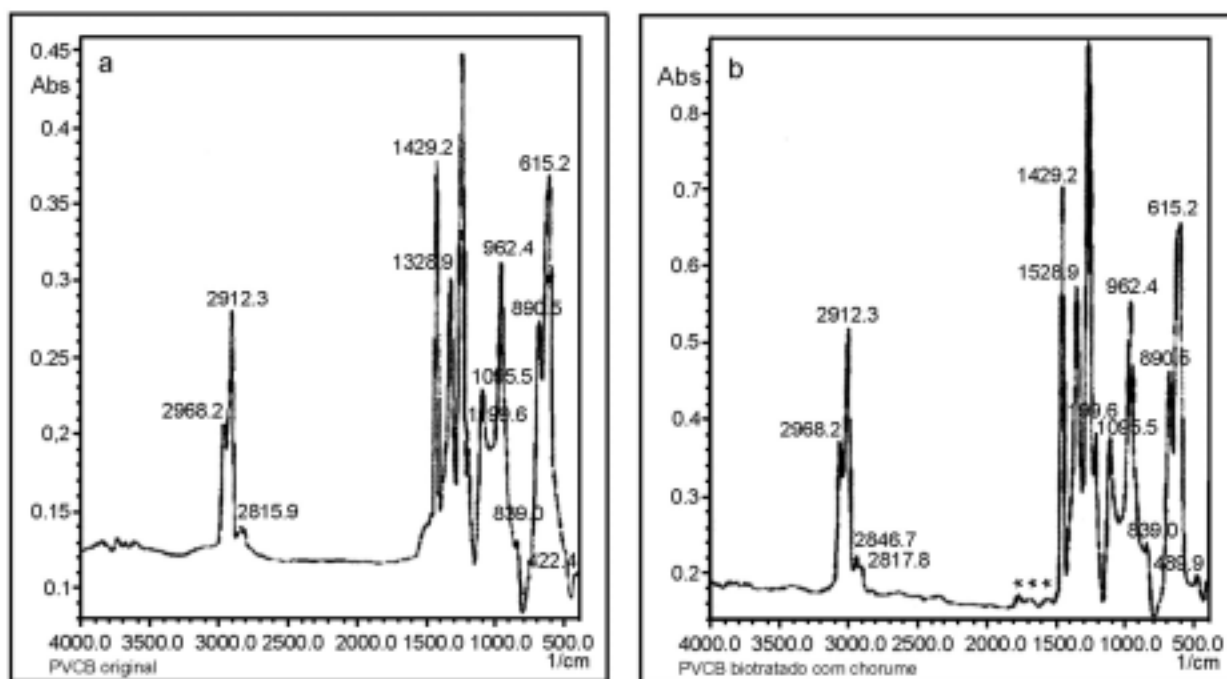
Fig. 1 - FTIR de Filmes de PVC biotratados com suspensão de chorume, em meio líquido de Sabouraud e meio mineral, durante 3 meses, à temperatura ambiente.
