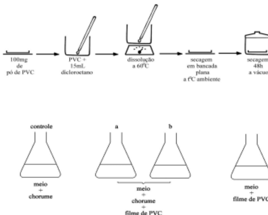
Esquema 1 - Preparo de filmes de PVC por evaporação de soluções de dicloroetano, a 60°C, com secagem à vácuo e Biotratamento por incubação dos filmes de PVC (duplicatas a,b) em meio Sabouraud líquido com suspensão de chorume, durante 3 meses, à temperatura ambiente.
